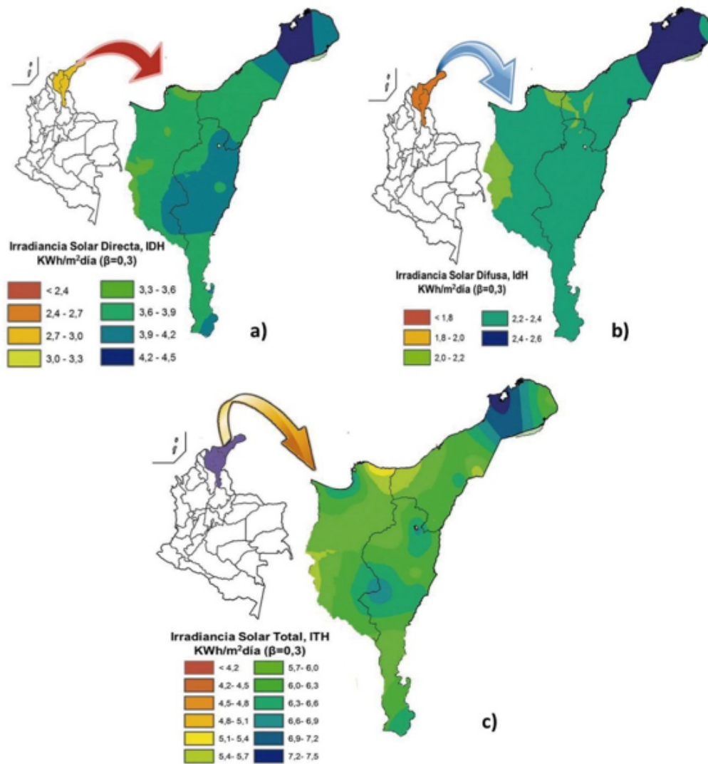
Figura 8. Mapa de Radiación Solar a) Directa b) Difusa c) Total (ITH KWh/m 2 día) promedio anual de la Zona de estudio para una atmósfera turbia (β=0,3) Fuente: Elaboración propia
