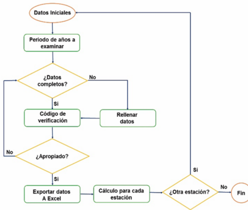
Figura 2. Algoritmo para el tratamiento de los datos meteorológicos suministrados por el IDEAM. Fuente: Elaboración propia.
