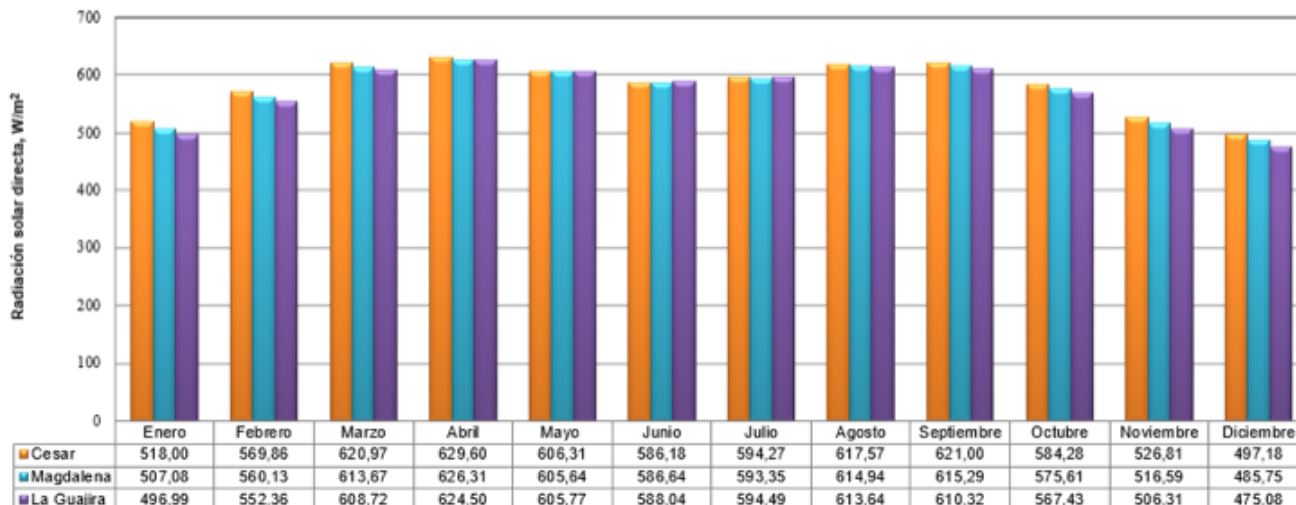
Figura 4. Promedio histórico mensual de la radiación solar directa de la zona de estudio teniendo en cuenta una atmósfera turbia (β=0,3).
