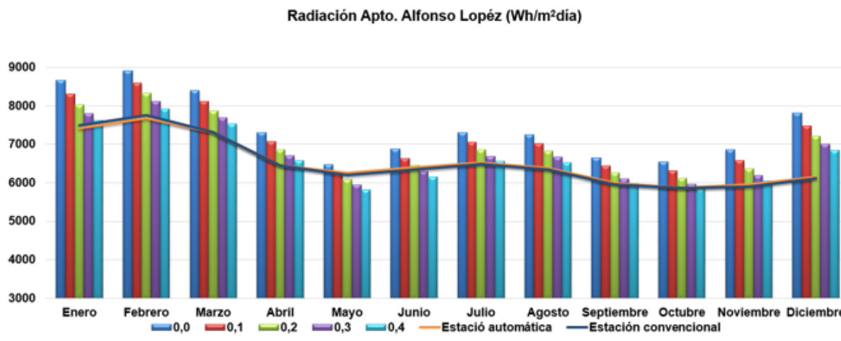
Figura 10. Comparación de la radiación calculada a través del modelo de Bird y Hulstrom con la medida a través de estaciones automáticas y convencionales de la estación Apto. Alfonso López (Valledupar, Cesar). Fuente: Elaboración propia
