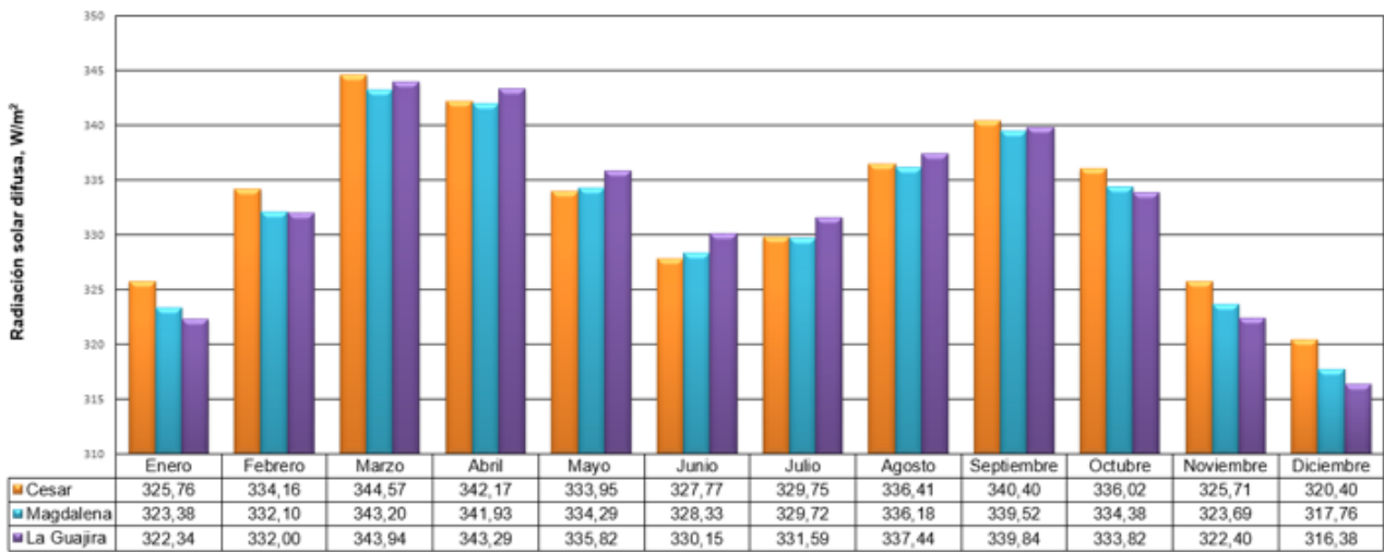
Figura 5. Promedio histórico mensual de la radiación solar difusa de la zona de estudio teniendo en cuenta una atmósfera turbia ( \beta=0,3 ). Fuente: Elaboración propia
